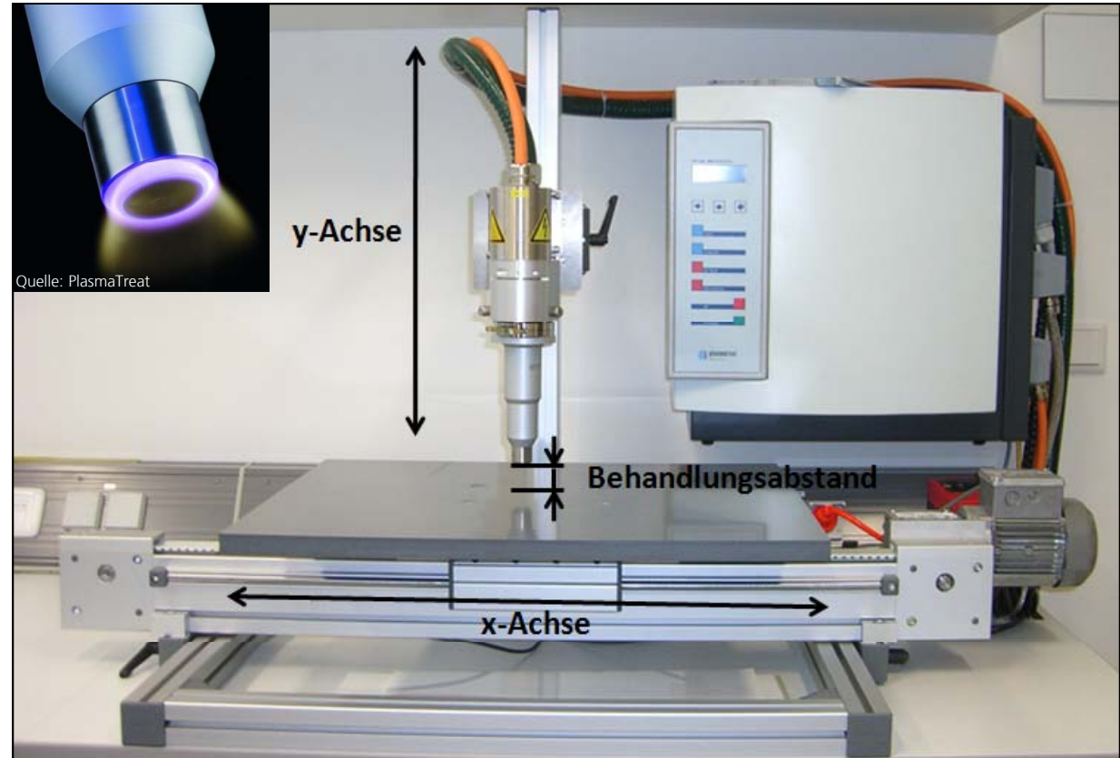
Plasma-Vorbehandlungsanlage mit Lineartisch, Plasmaustritt an Rotationsdüse
